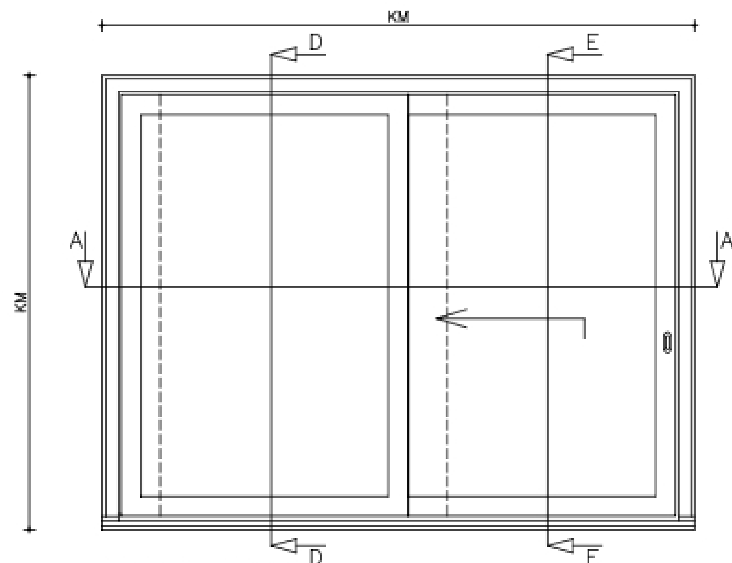
BUITENAANZICHT
