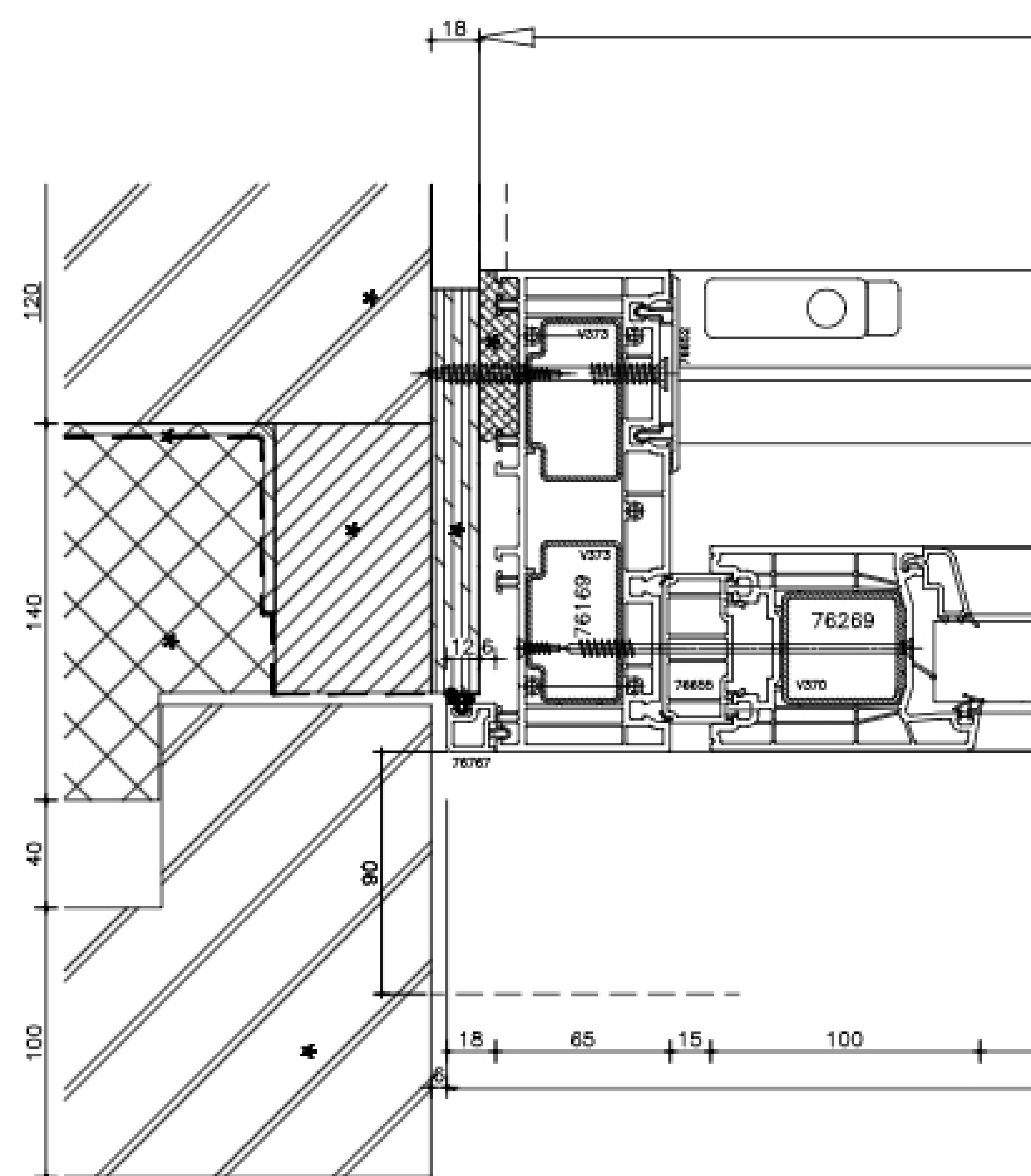
DOORSNEDE A-A
