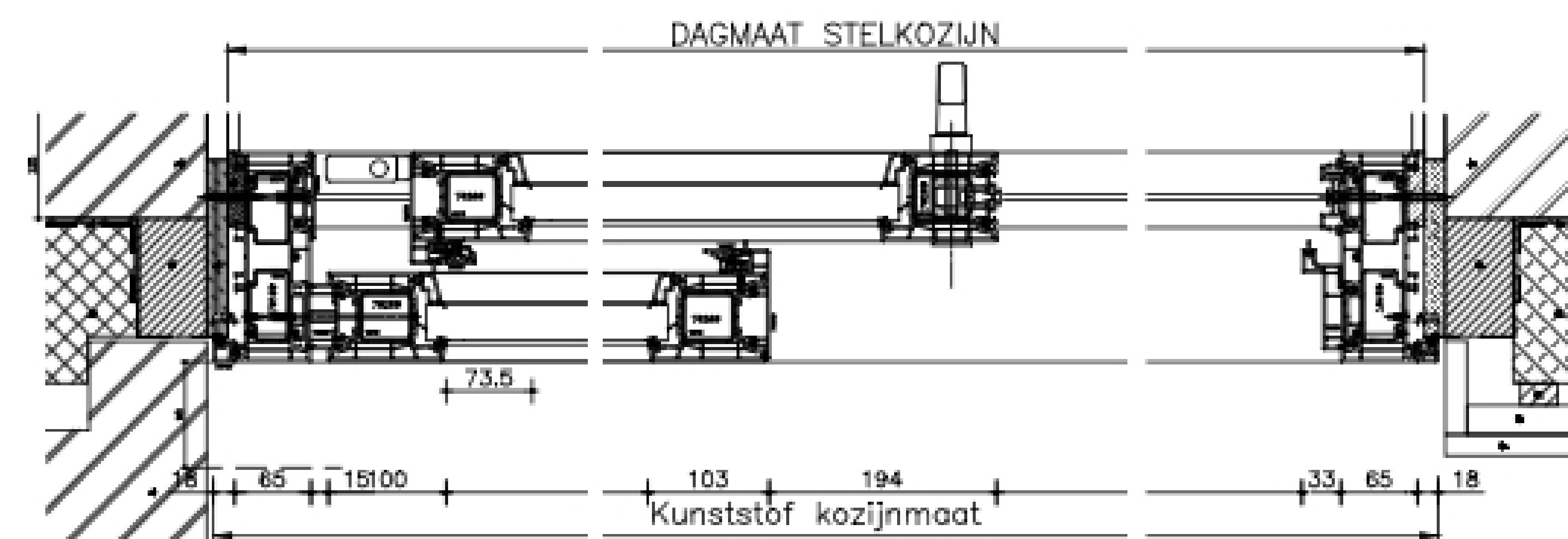
DOORSNEDE A-A DEUR IN OPENSTAND
